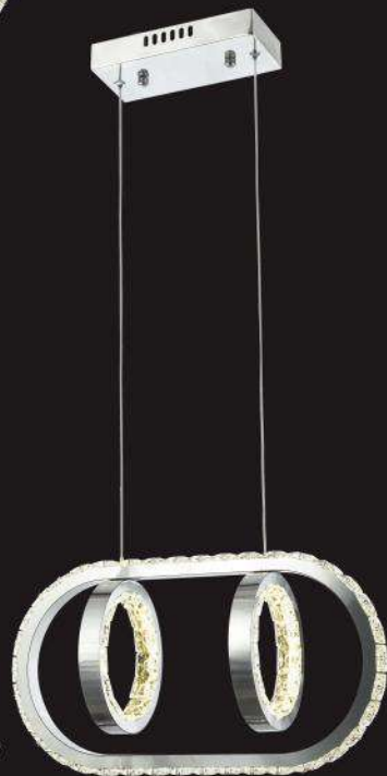
L7814-2 L470×W250×H1200mm Chrome 3000-4500-6000K 44W
